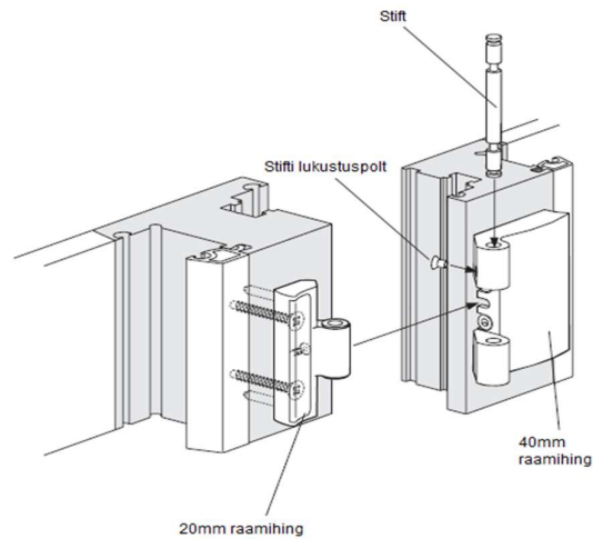
Joonis 19. ROTO Patio 6080 hingede kinnitamine, raam
