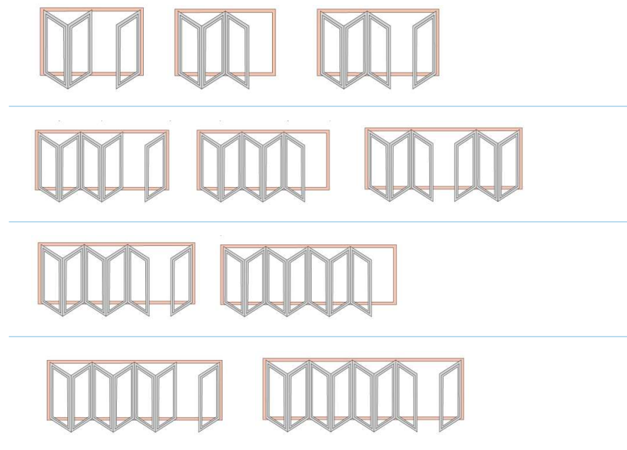
Joonis 16. ROTO Patio 6080 avanemise skeemid
