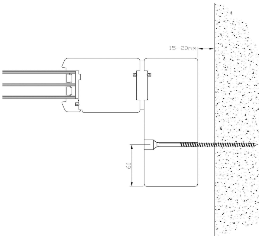
Joonis 14. Paraleellükandukse lengi fikseerimine (vert)
