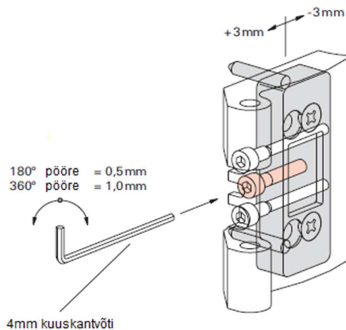
Joonis 20. ROTO Patio 6080 reguleerimine kuuskantvõtmega
