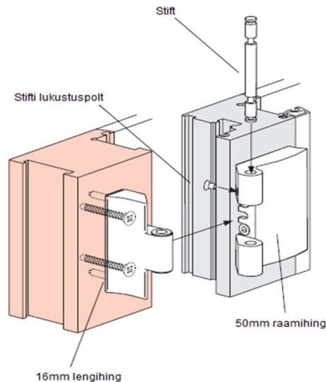
Joonis 18. ROTO Patio 6080 hingede kinnitamine, leng
