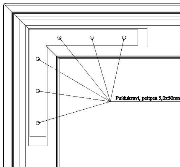
Joonis 25. Lengide nurgaühenduse kinnitamine
