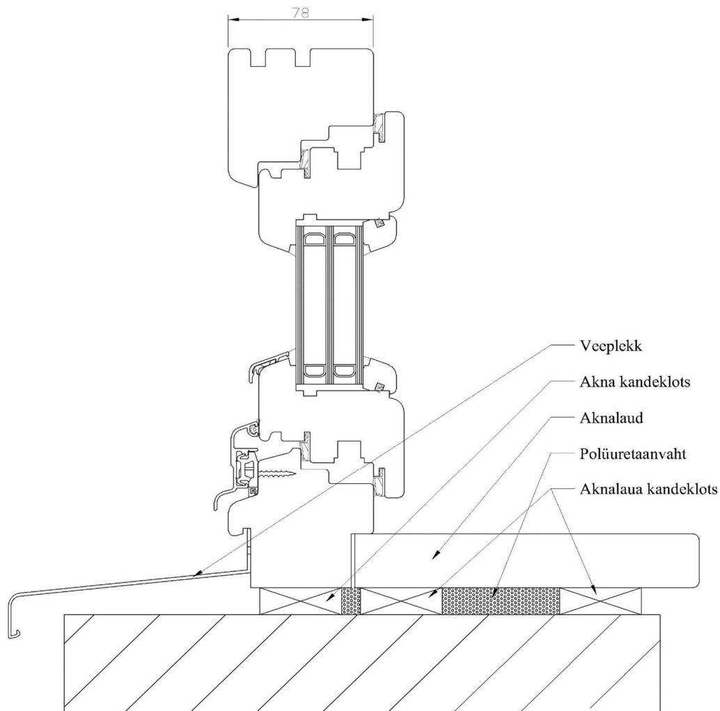
Joonis 23. Aknaalaua ja veepleki paigaldus
