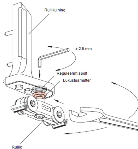
Joonis 21. ROTO Patio 6080 reguleerimine lehtvõtmega
