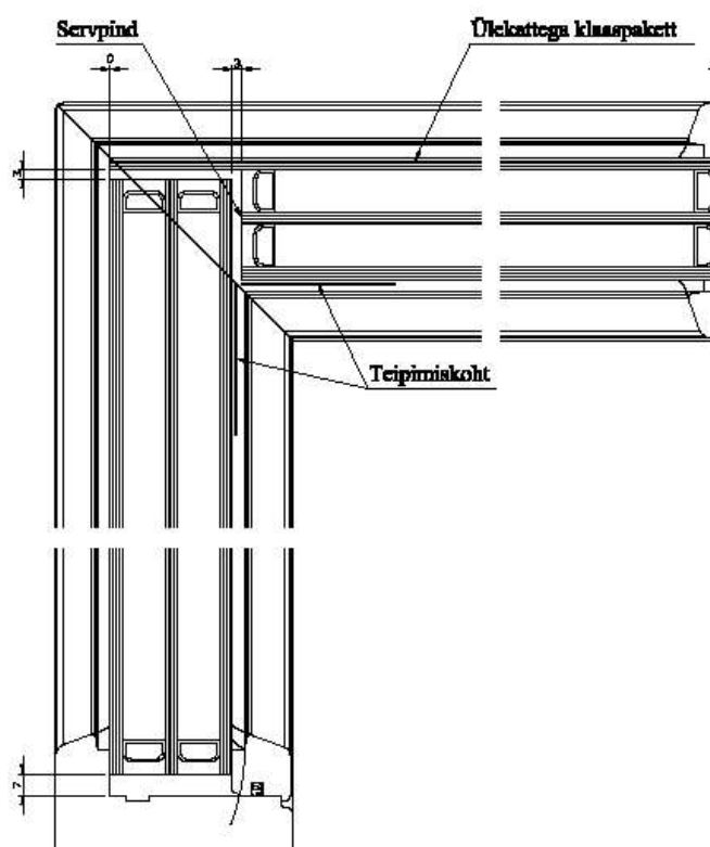
Joonis 26. Ülekattega klaaspaketi nurgaühendus
