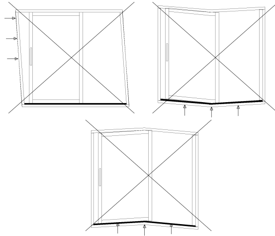
Joonis 15. Vale paraleellükandukse paigaldus
