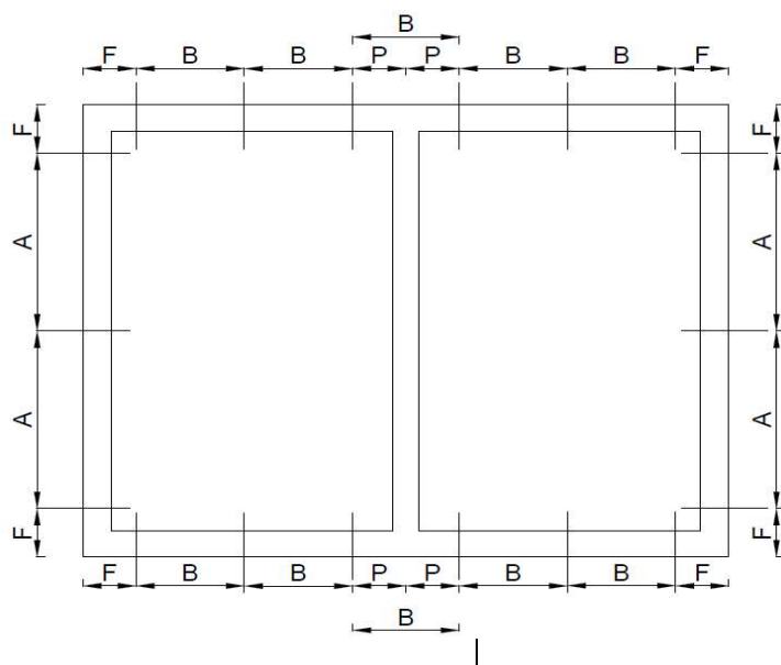
Joonis 5. Kinnituspunktide asetus
