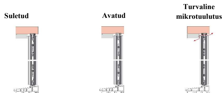
Joonis 15. ROTO Patio Life tööpõhimõte
