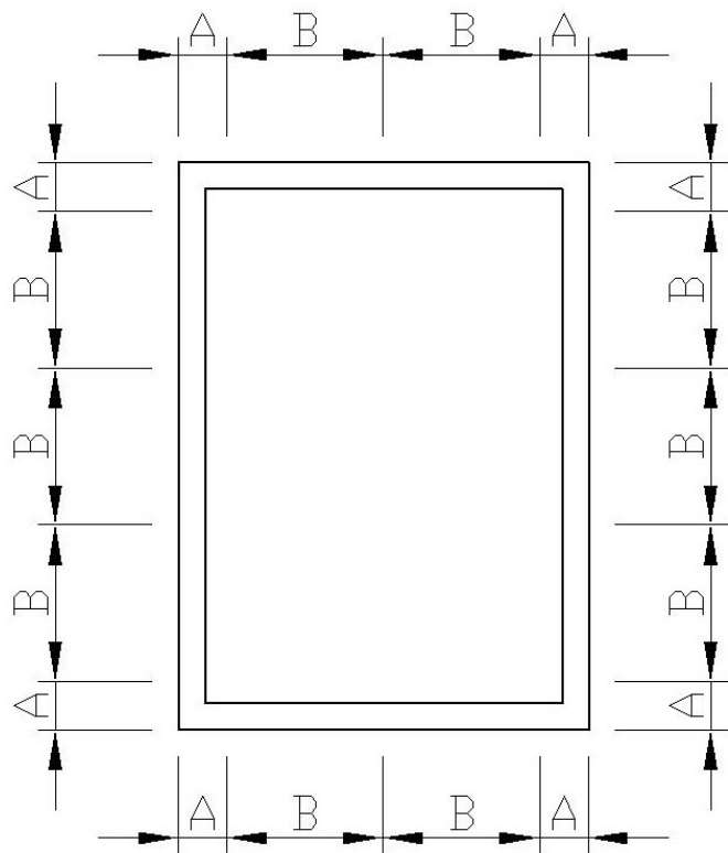
Joonis 22. Tuletõkkeakna tugiklotside ja kinnituspunktide asetuse.
