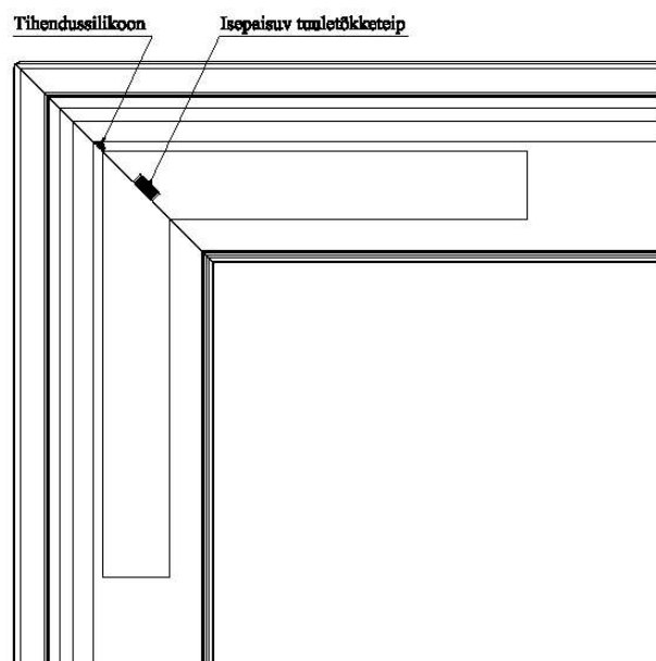
Joonis 24. Lengide nurgaühenduse tihendamine
