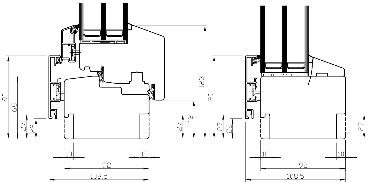
B - B
