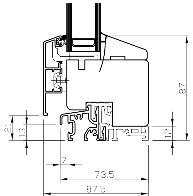
B - B
