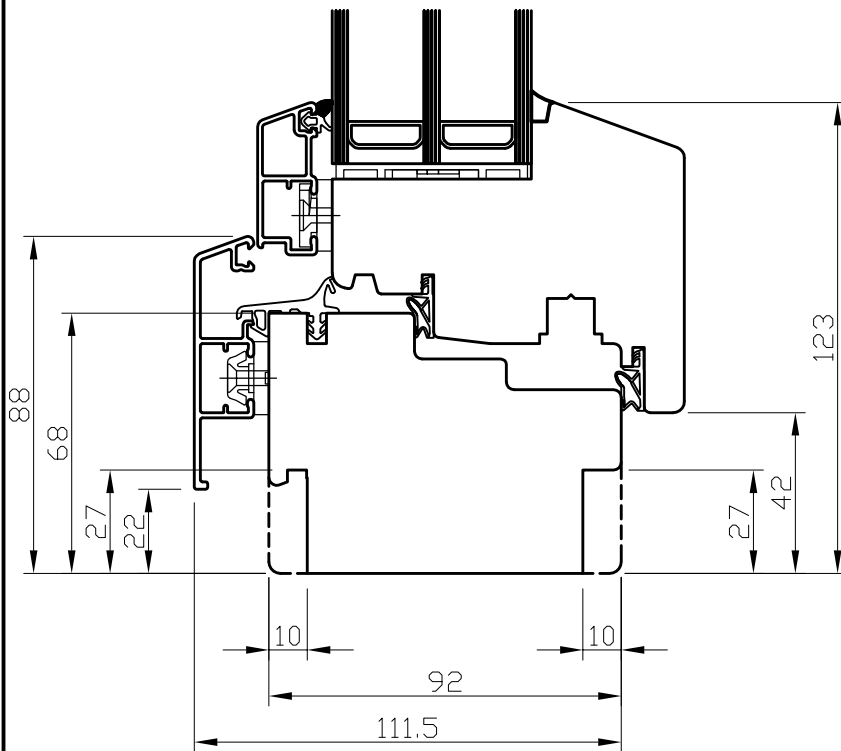
A - A
